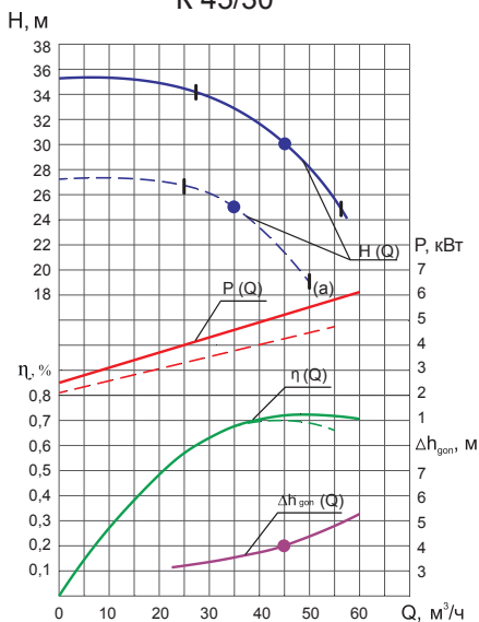
K 45/30
