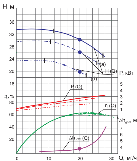
1K 20/30
