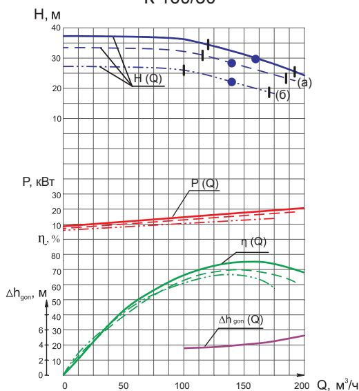
K 160/30
