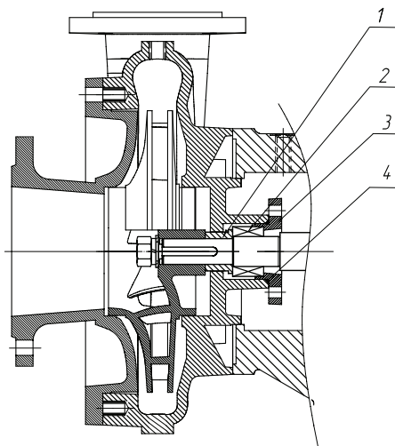
Рисунок 1.2. Насос консольный 1К и К с одинарным торцевым механическим уплотнением типа 5
