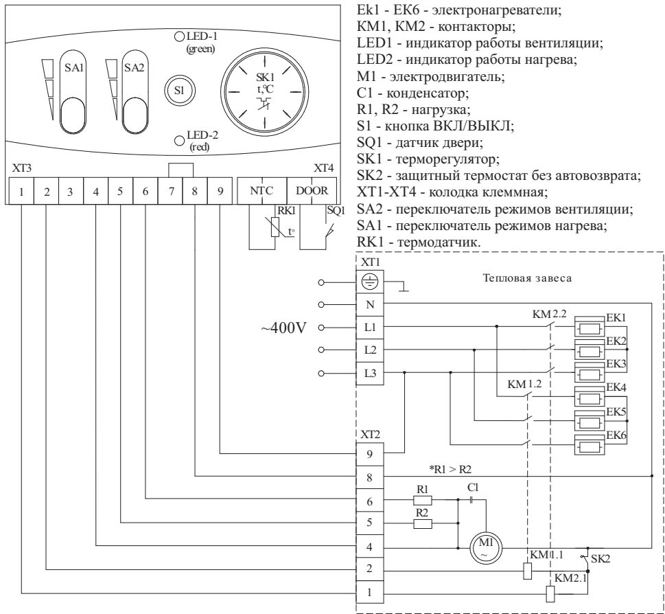
Рисунок 17. Схема электрическая принципиальная завес KVC-D10E12 -31, KVC-D10E18 -31, KVC-D15E12 -31, KVC-D15E18 -31 и KVC-D15E24 -31
