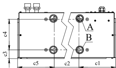
ГОРИЗОНТАЛЬНАЯ УСТАНОВКА к потолку на шпильки
