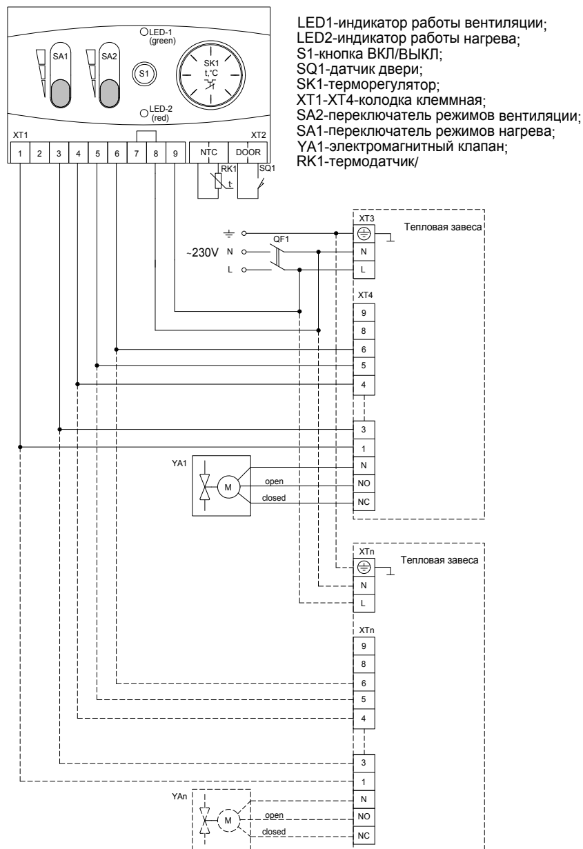
Рисунок 17. Групповая схема подключения занес к контроллеру KRC-32
