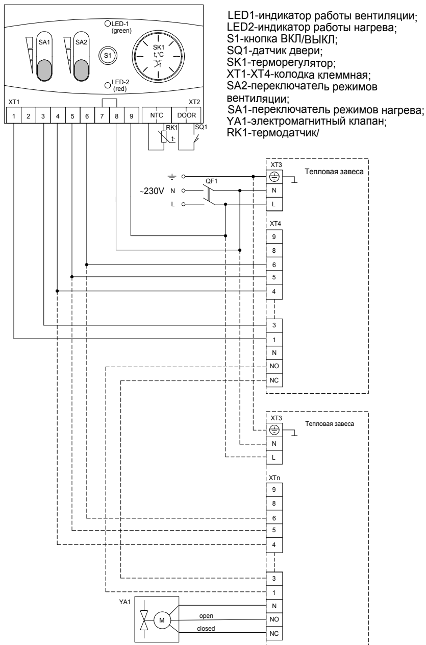
Рисунок 18. Групповая схема подключения занес к контроллеру KRC-32
