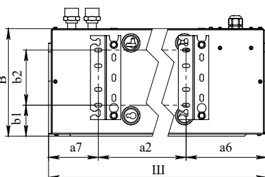
РАЗМЕРЫ КРОНШТЕЙНА
