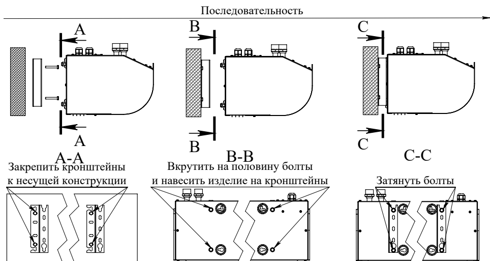
Рисунок 12. Схема крепления завесы горизонтально над проемом к стене с помощью кронштейнов.
