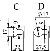
Рисунок 9. Габаритные и крепежные размеры
