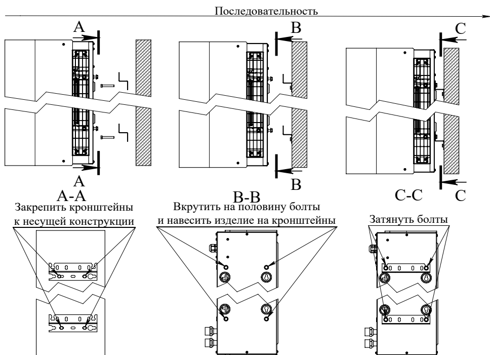
Рисунок 13. Схема крепления завесы вертикально к стене с помощью кронштейнов.
