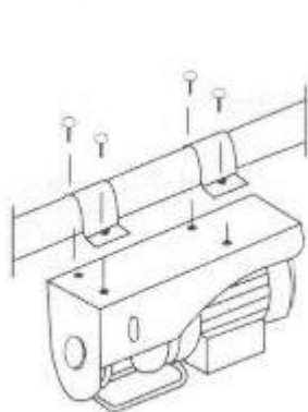
Рис.3 - Установка тали
