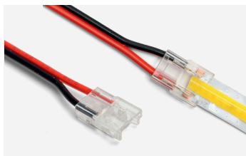
WLS-A-07 Коннектор выводной для ленты COB
