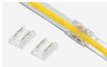
WLS-A-06 Коннектор последовательный для ленты COB
