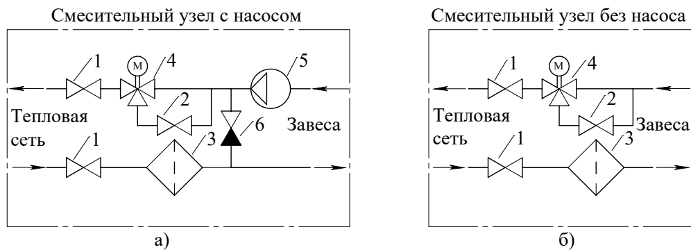
Рисунок 20. Схемы смесительных узлов
