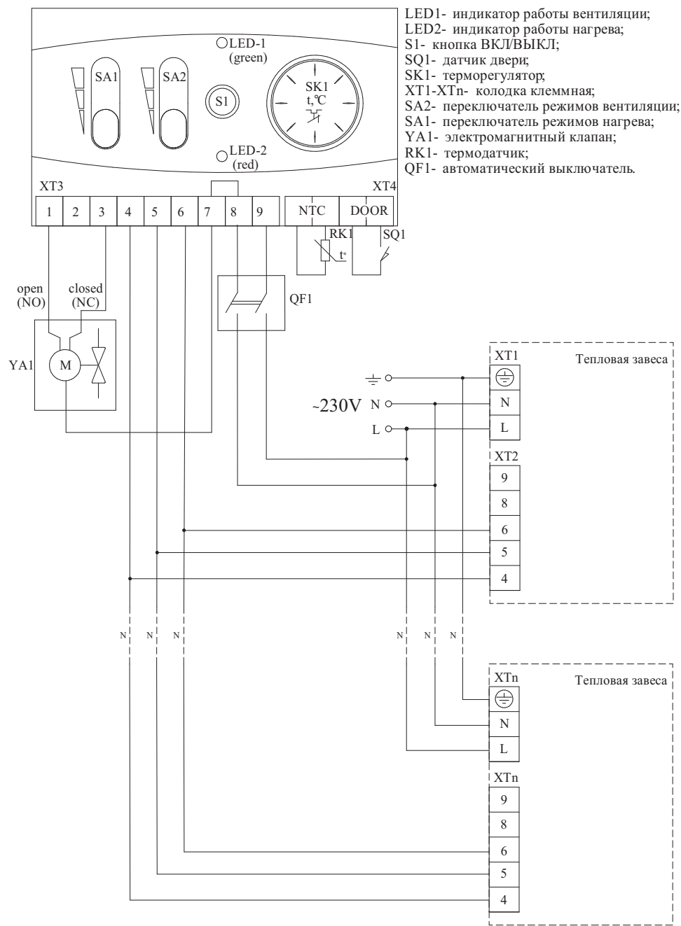
Рисунок 17. Групповая схема подключения занес к контроллеру KRC-32
