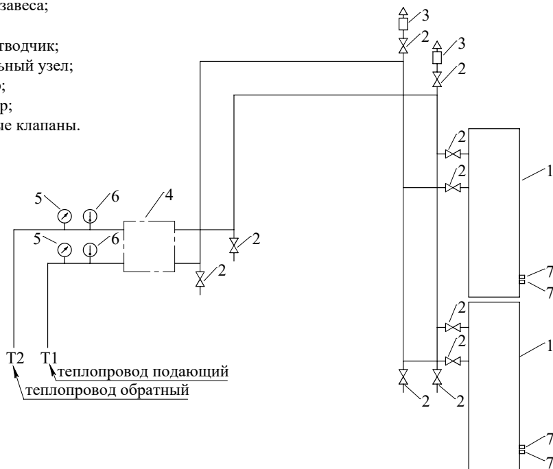
Рисунок 18. Схема подключения к тепловой сети вертикально расположенных завес
