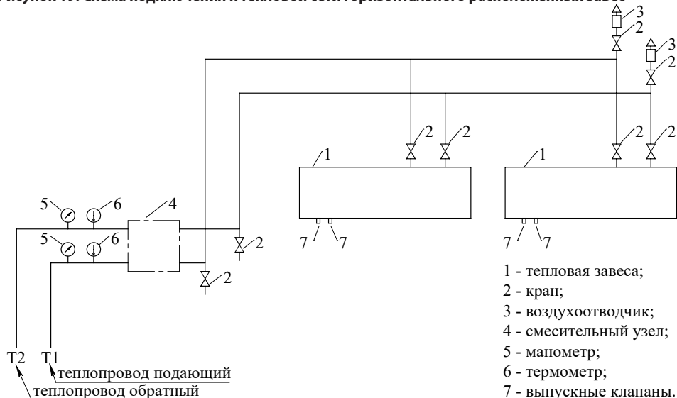
Рисунок 19. Схема подключения к тепловой сети горизонтального расположенных завес
