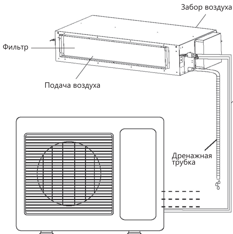
Внутренний блок (типоразмер 18/24/36)
