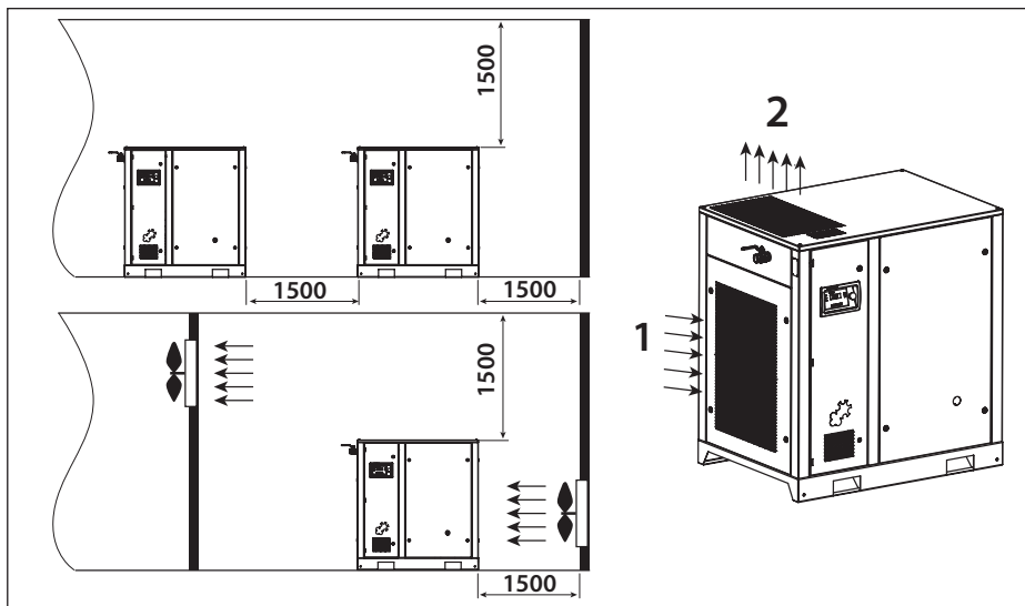
Bild 3.4 Installationsvorschlag D30-D55
