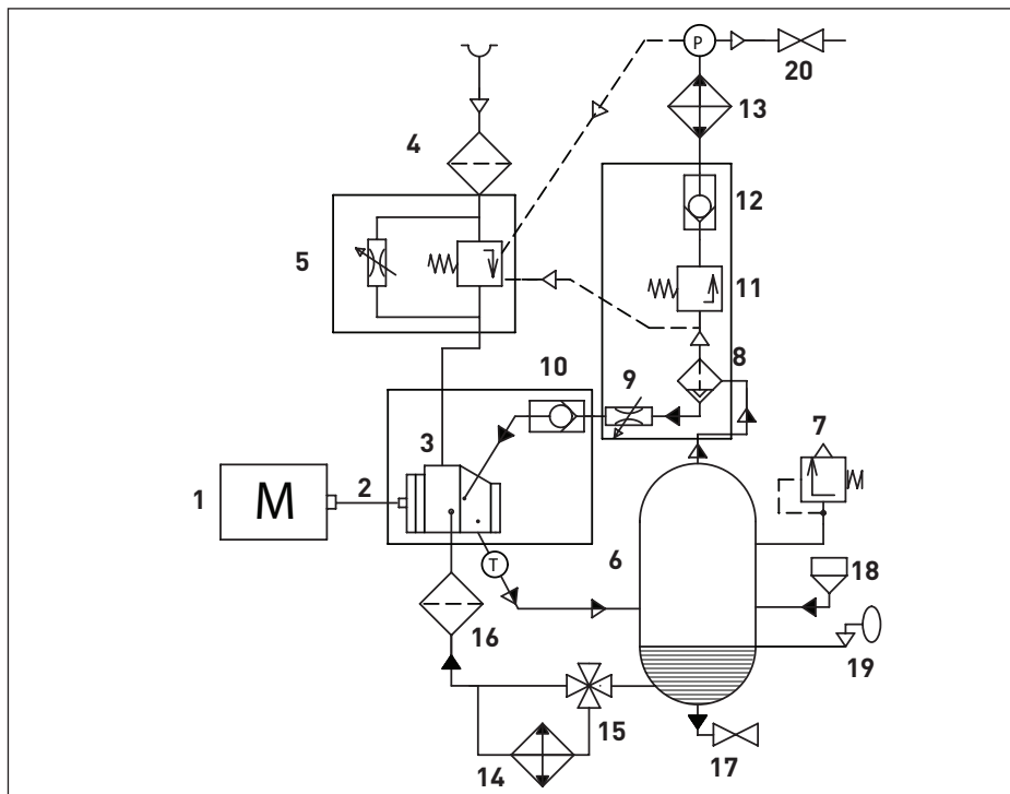
Bild 2.3 Ablaufdiagramm D30–D55
