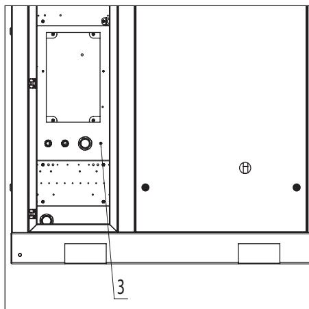
Bild 3.6.2 Stromkabel Klemmverbindungen
