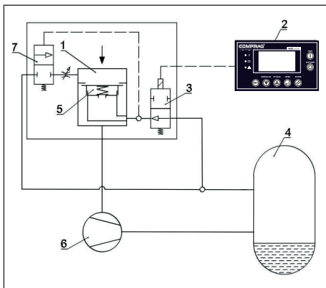
Bild 2.5 Pneumatikplan
