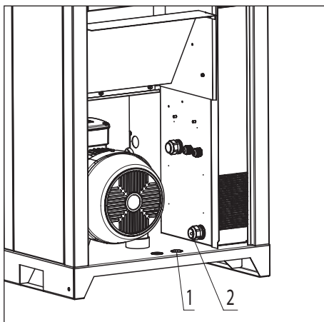
Bild 3.6.1 Stromkabelverbindung
