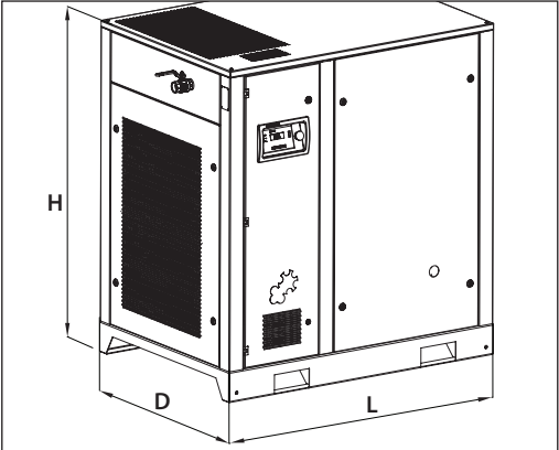
Bild 3.2 Abmessungen D30-D55
