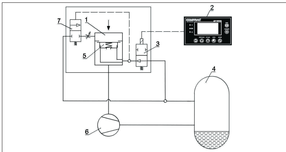
Рис. 2.5 Система регулировки
