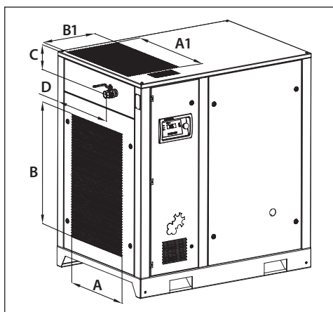
Bild 3.3 Einbauabmessungen D30-D55
