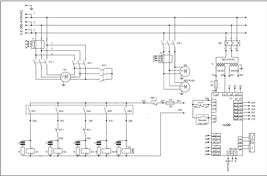
Bild 2.6 Elektro-Schaltplan D30-D55
