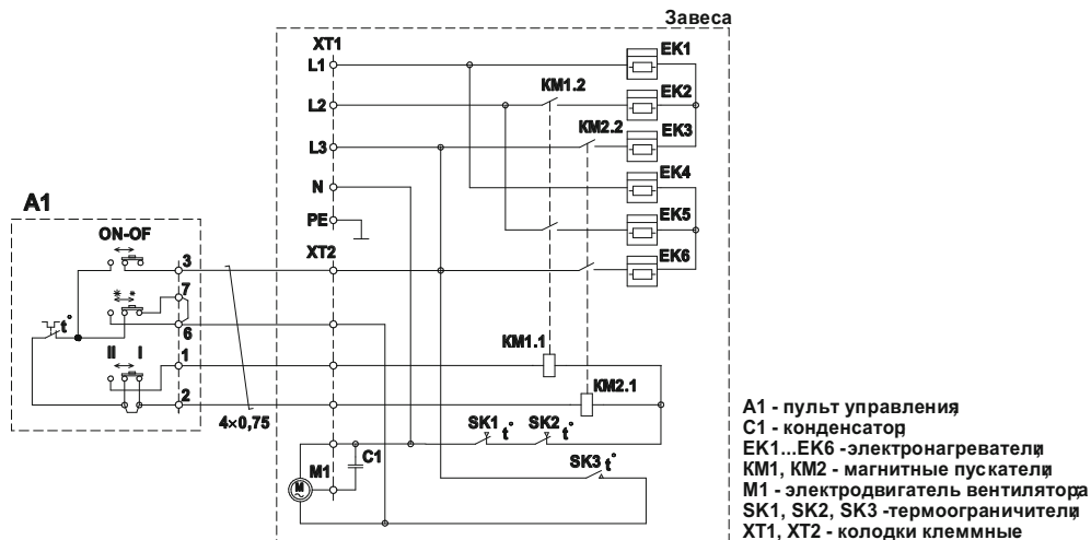
Рис 2. Схема электрическая
