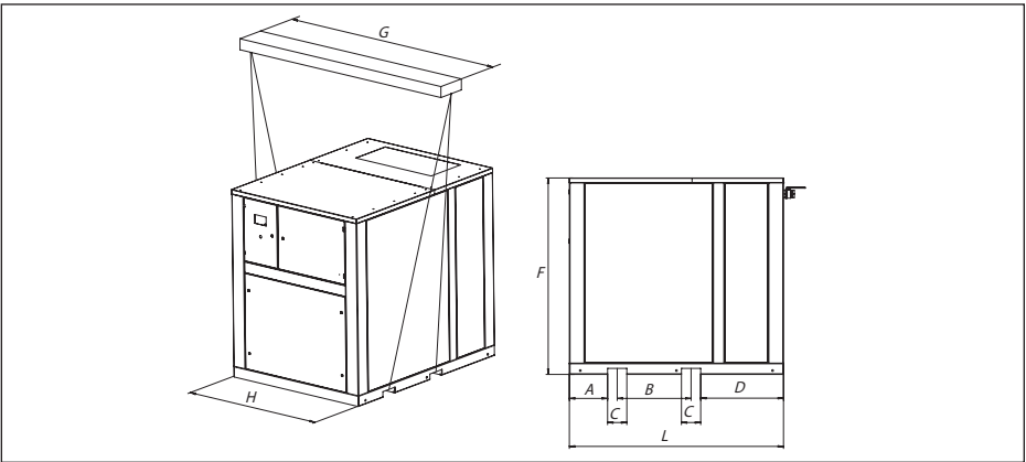
Рис. 3.1 Схема для такелажных работ A75-90
