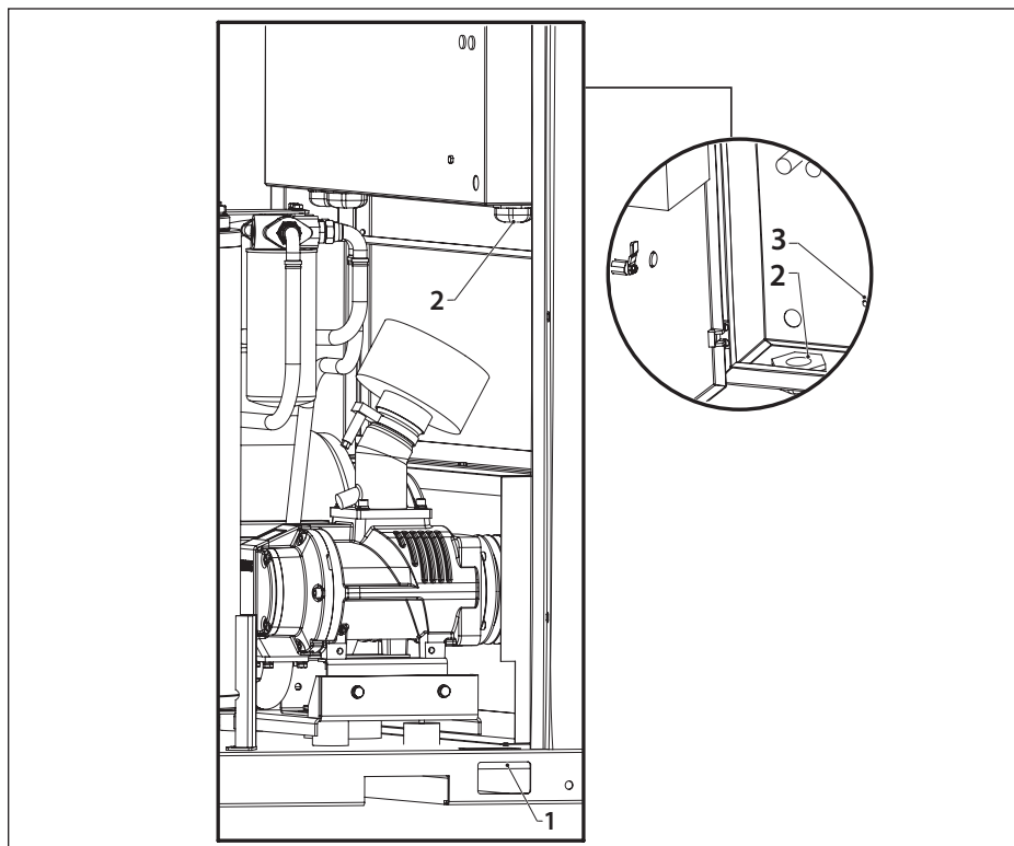
Bild 3.5 Stromkabelverbindung
