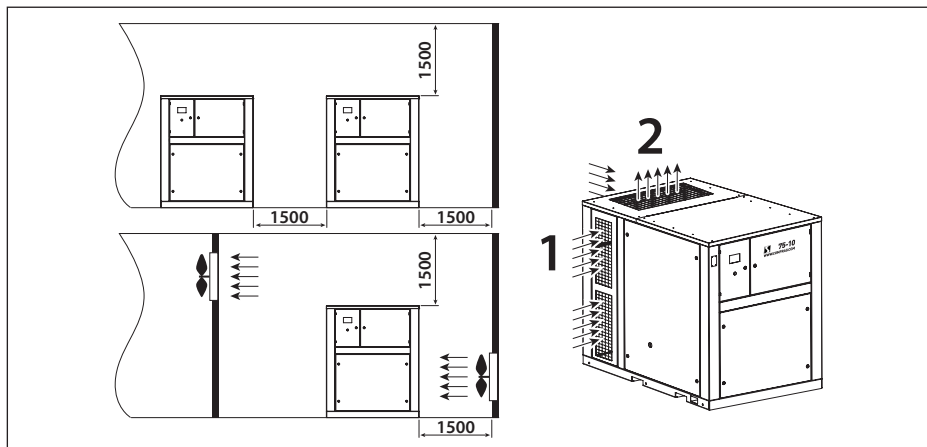
Рис. 3.3 Схема установки компрессора A75-90
