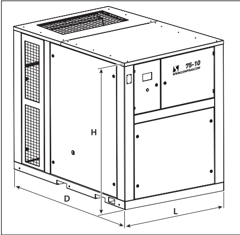
Bild 3.2 Abmessungen A75–90
