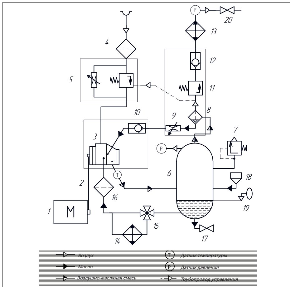
Рис. 2.3 Схема пневматическая А75-90
