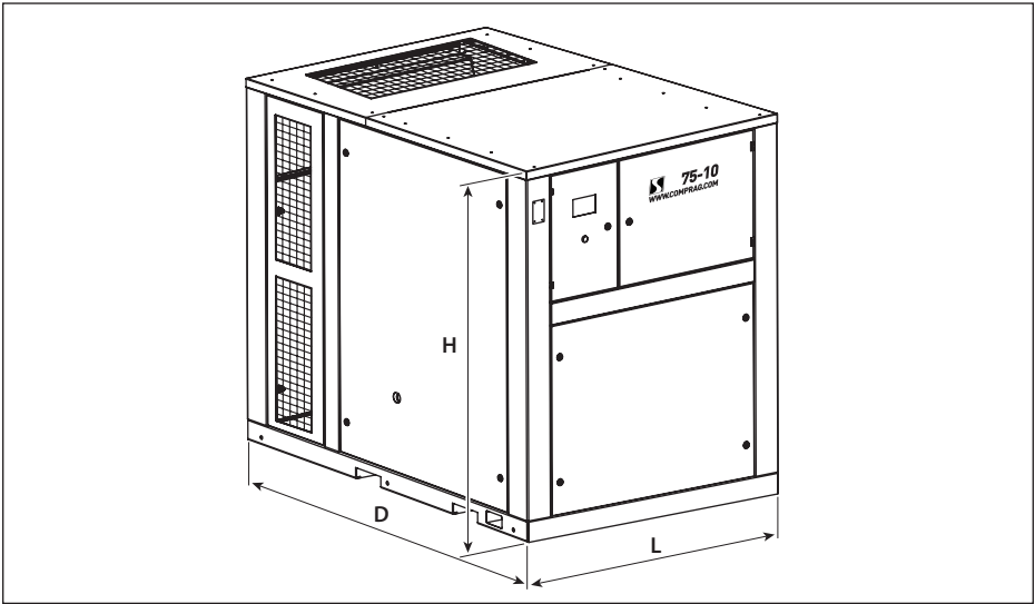
Рис. 3.2 Габаритные размеры А75 – 90
