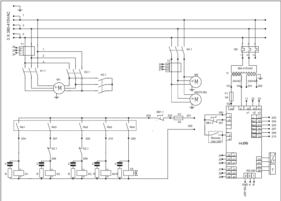
Bild 2.6 Elektro-Schaltplan A75-90
