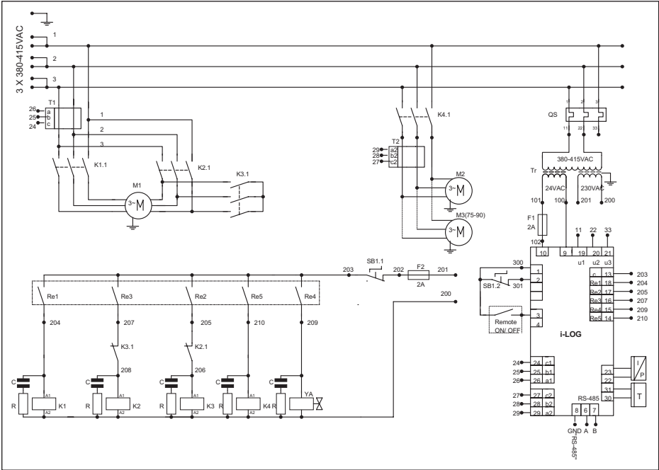
Fig. 2.6 Схема электрическая A75-90
