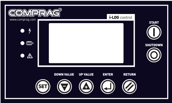
Bild 4.1.1 Bedienfeld i-Log
