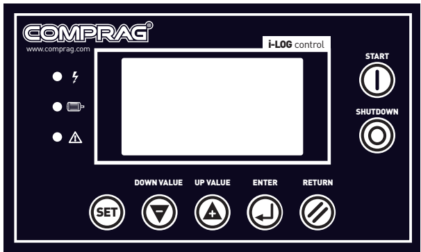
Bild 4.1.1.1 Bedienfeld i-Log
