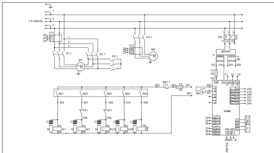
Bild 2.6 Elektro-Schaltplan A30-A55
