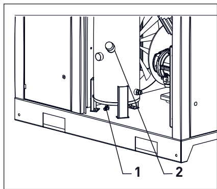
Рис. 5.4.1 Замена масла
