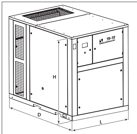
Bild 3.2 Abmessungen AV75–90
