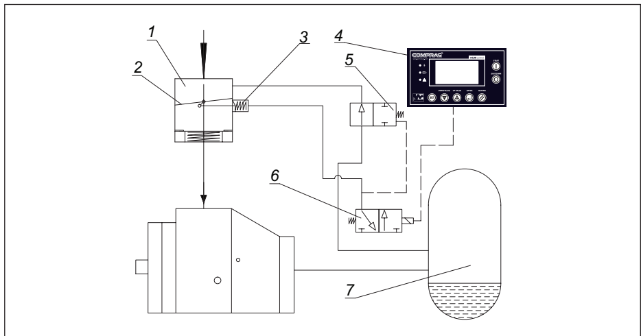
Bild 2.5 Pneumatikplan
