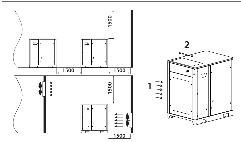
Bild 3.3 Installationsvorschlag AV30–55
