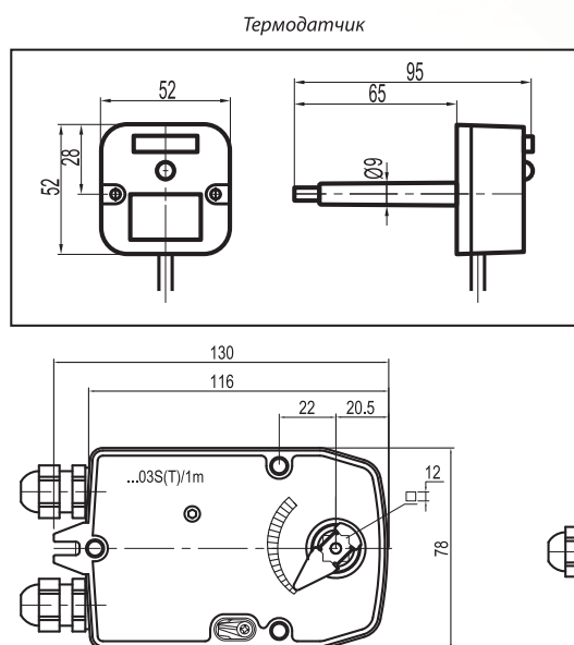
РАЗМЕРЫ мм
