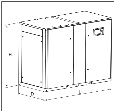
Bild 3.2 Abmessungen DV75–90
