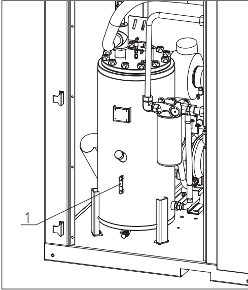
Bild 5.2 Ölstandsüberwachung
