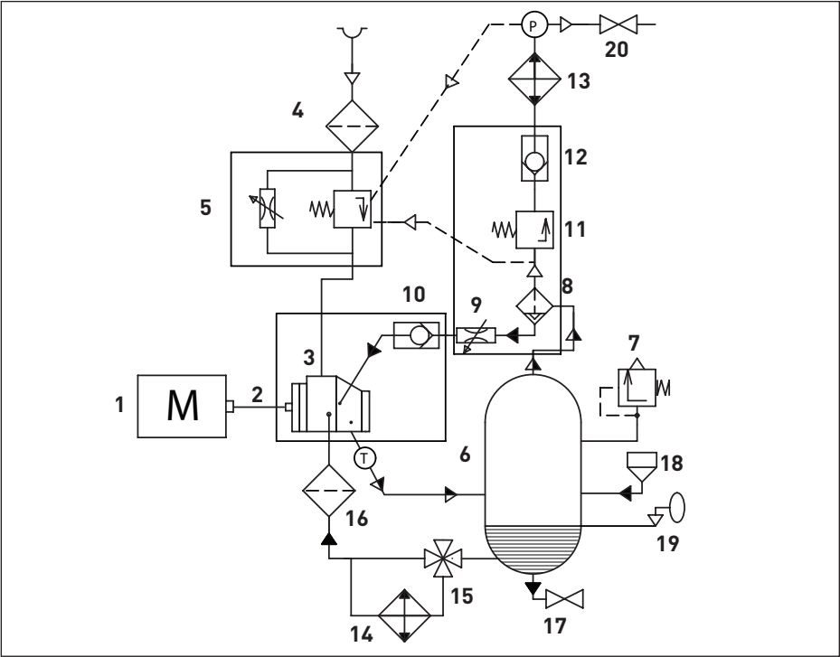
Bild 2.3 Ablaufdiagramm DV30-55
