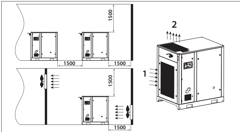
Bild 3.3 Installationsvorschlag DV30–55
