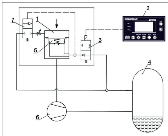
Bild 2.5 Pneumatikplan
