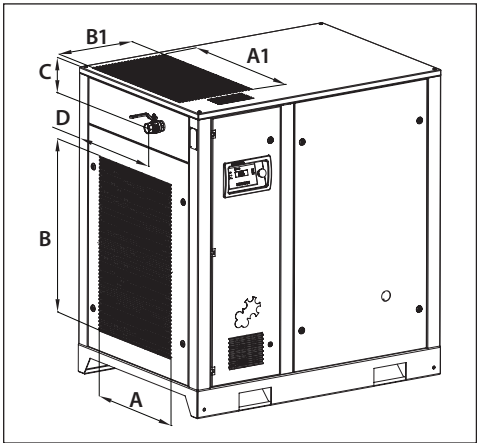
Bild 3.3 Einbauabmessungen DV30-55
