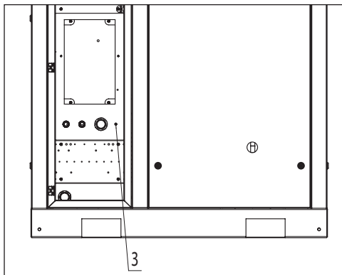
Bild 3.5.2 Stromkabel Klemmverbindungen
