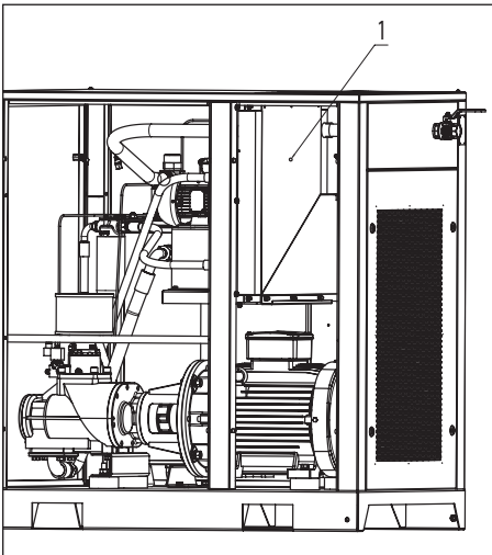
Bild 5.7 Wärmeaustauscher reinigen
