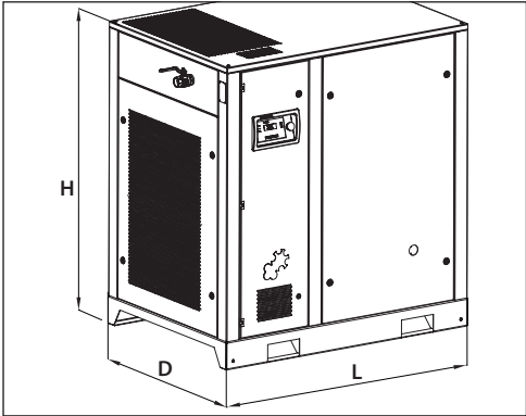
Bild 3.2 Abmessungen DV30–55
