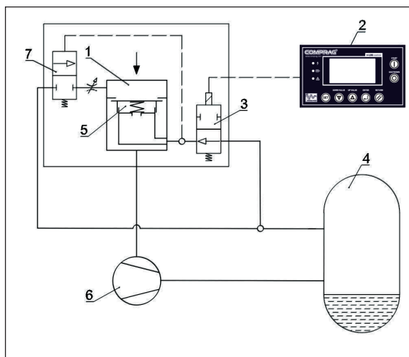
Рис. 2.5 Система регулировки
