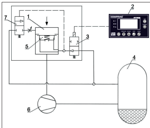
Bild 2.5 Pneumatikplan
