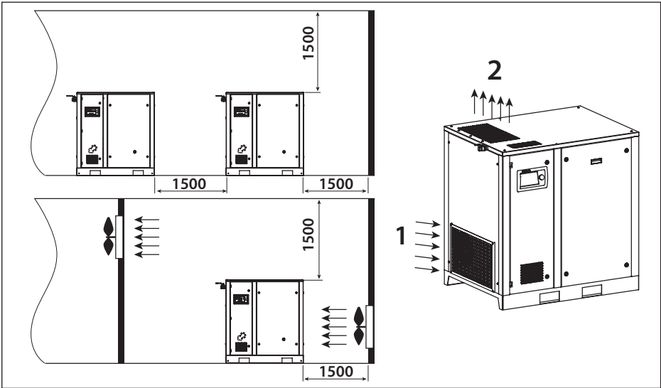
Bild 3.4 Installationsvorschlag DV11 – DV22
