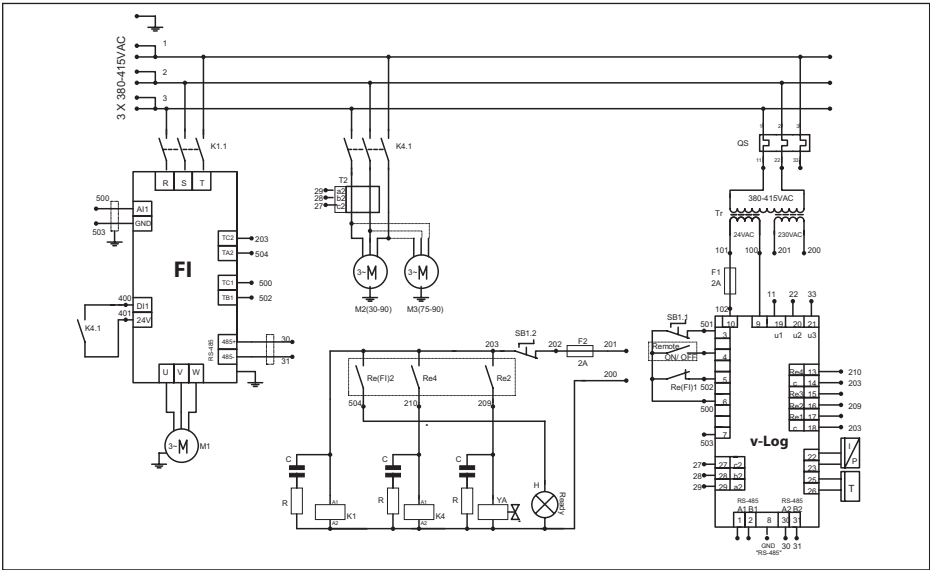
Bild 2.6.1 Elektro-Schaltplan DV11 – DV22
