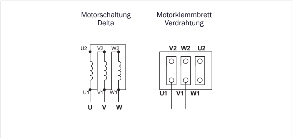
Bild 2.6.2 Elektrischer Schaltplan für DV11 – DV22
