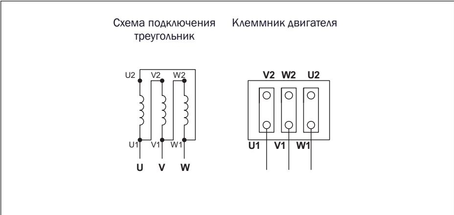
Рис. 2.6.2 Схема подключения двигателя DV11 – DV22
