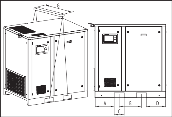
Bild 3.1 Heben und Transportieren DV11 – DV22
