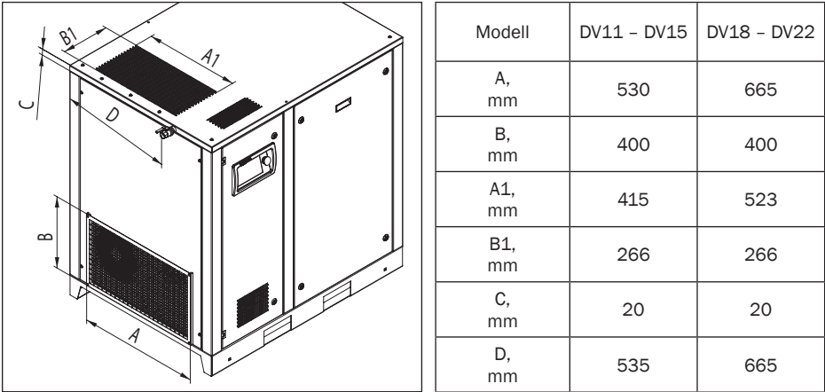
Bild 3.3 Einbauabmessungen DV11 – DV22
