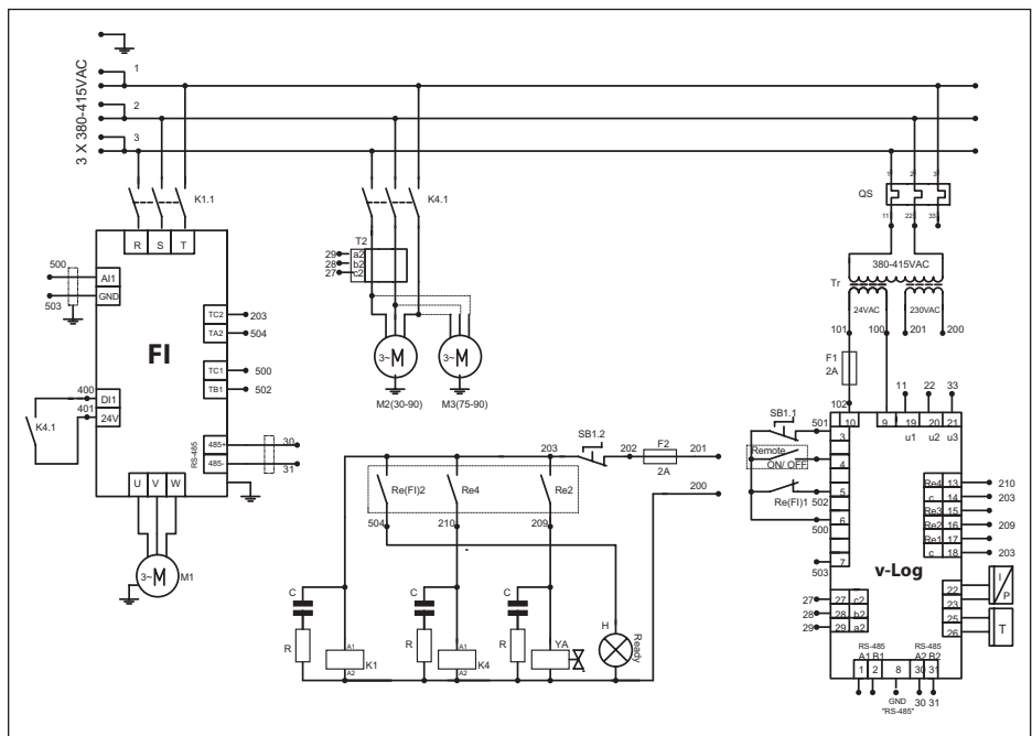
Рис. 2.6.1 Схема электрическая DV11 – DV22
