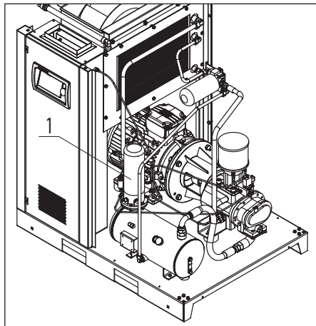
Bild 5.5.2 Austausch des Luft/ Öl-Separator DV18 – DV22
