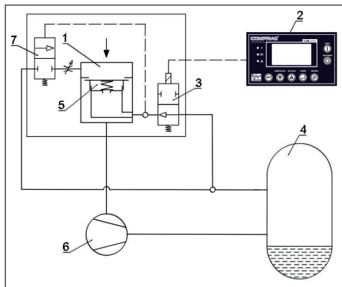
Рис. 2.5 Система регулировки
