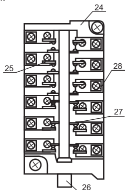
Рисунок 8. Электромагнит контакторов КТП6600Н
