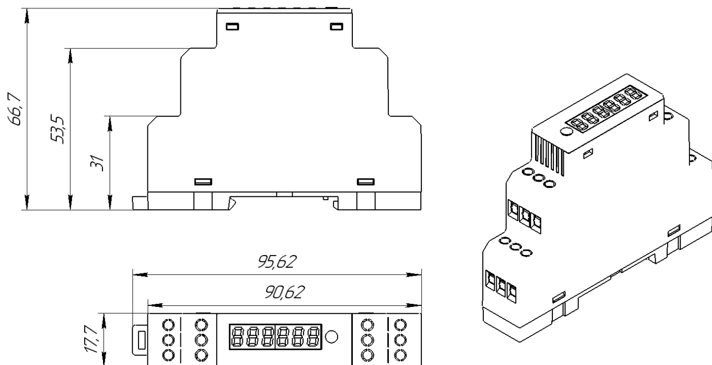
Рис. 1. Установочные размеры
