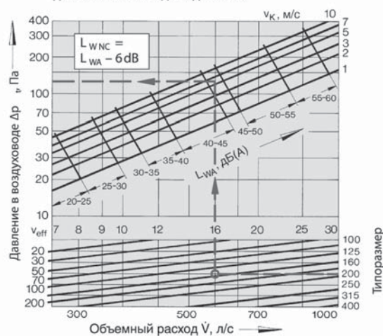
9 Звуковая мощность и потеря давления для бокового подсоединения
