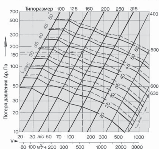
8 Мощность звука и падение давления для аксиального подсоединения KV поворотн. сопла
