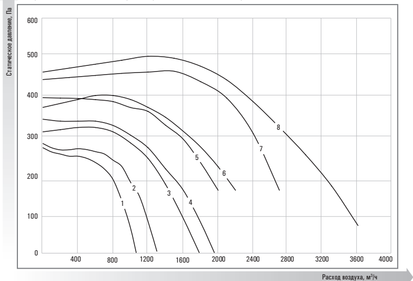
Аэродинамические характеристики вентиляторов
