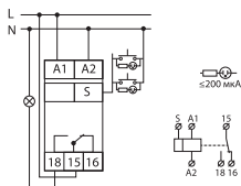
Рисунок 2. Схемы подключения реле к сети
