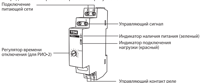
Рисунок 4. Передняя панель реле RIO-1 и RIO-2
