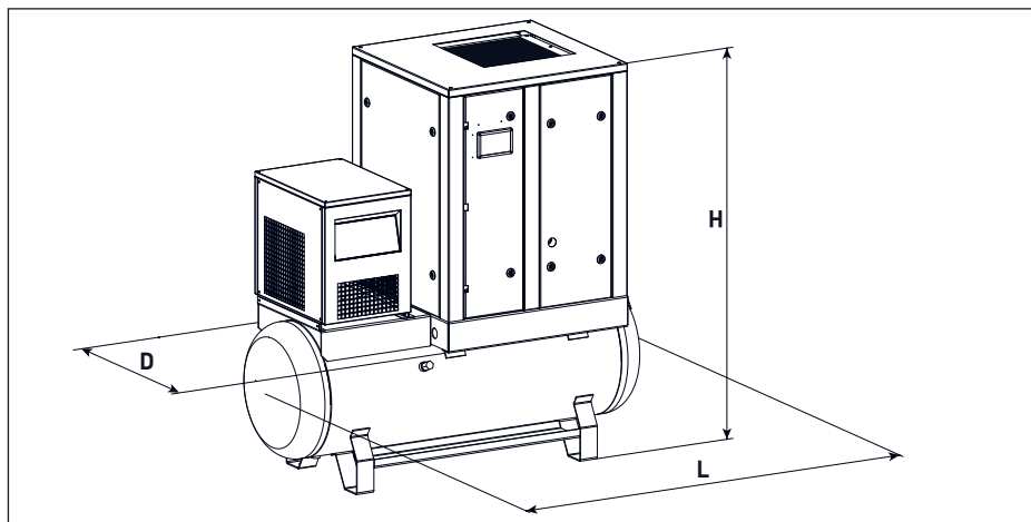
Bild 3.2.2 Abmessungen AR/FR..,ARD/FRD..
