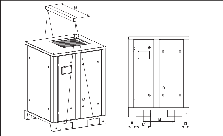
Рис. 3.1.1 Схема для такелажных работ A/F..
