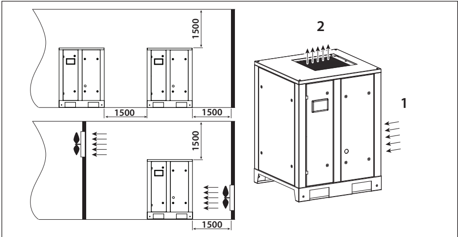
Bild 3.3.1 Installationsvorschlag A/F..
