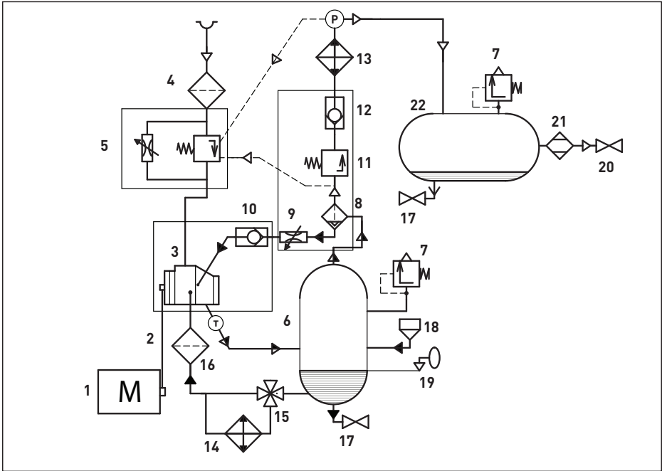
Bild 2.3.2 Ablaufdiagramm AR/FR..,ARD/FRD..
