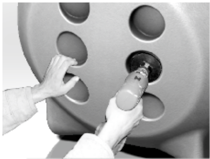
Рис. 10 Сверление отверстия для установки ЗПТ
