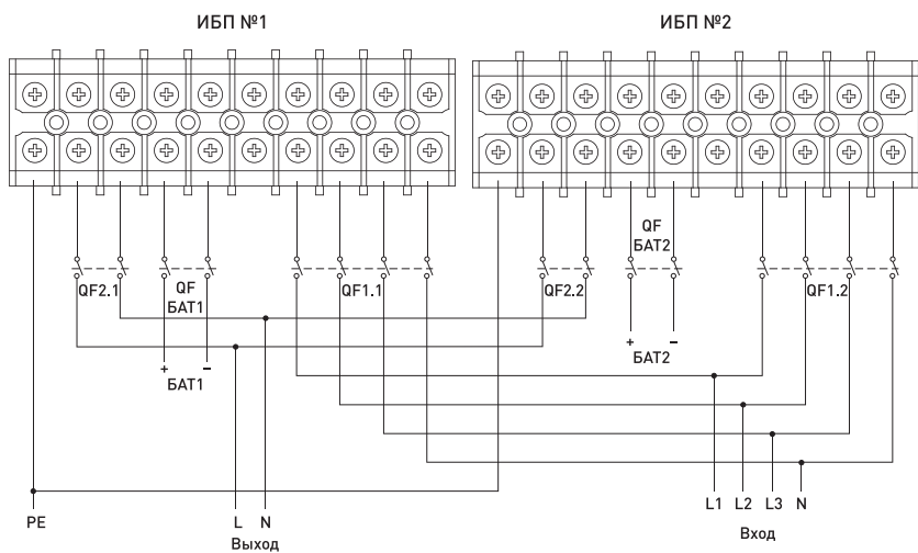
Рисунок 5 – Схема параллельного подключения ИБП 3:1
