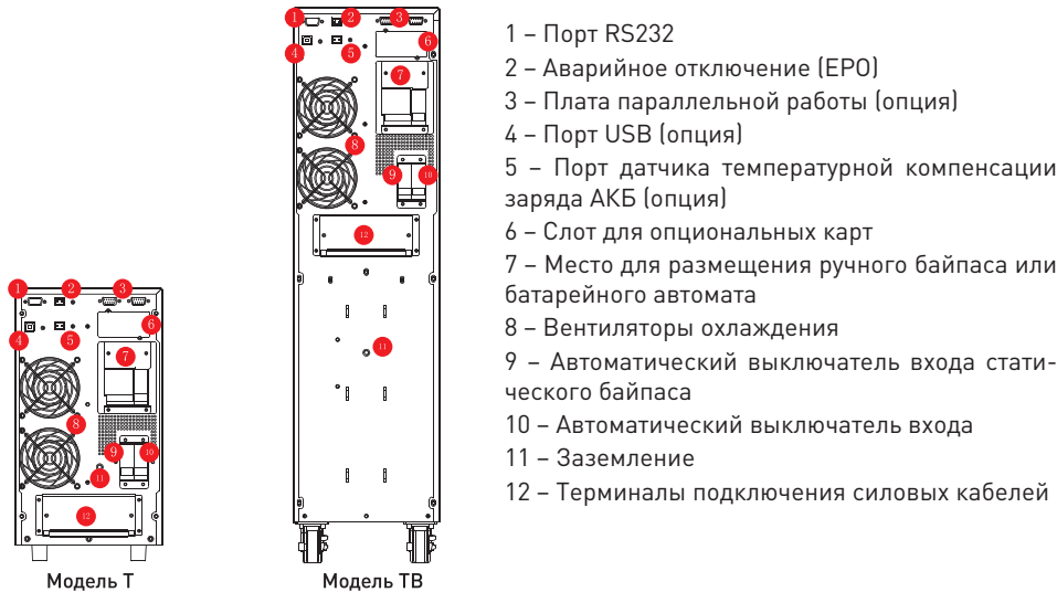
Рисунок 2 – ИБП, вид сзади. Условные обозначения:
