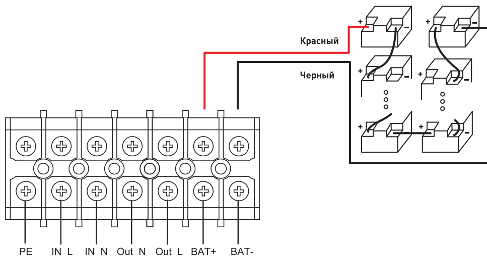
Рисунок 8 – Схема подключения внешних аккумуляторных батарей к ИБП
