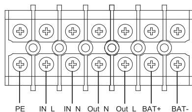
Рисунок 3 – Клеммная колодка ИБП
