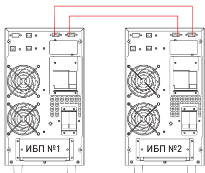
Рисунок 6 – Подключение коммуникационных кабелей 2х ИБП
