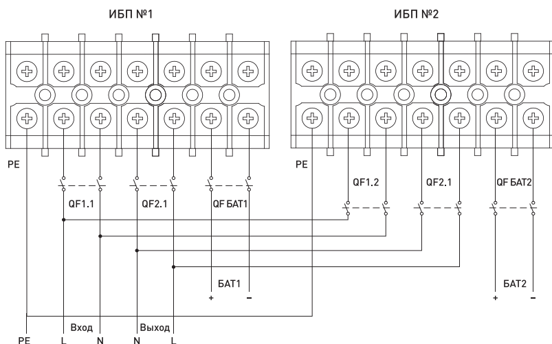
Рисунок 4 – Схема параллельного подключения ИБП 1:1
