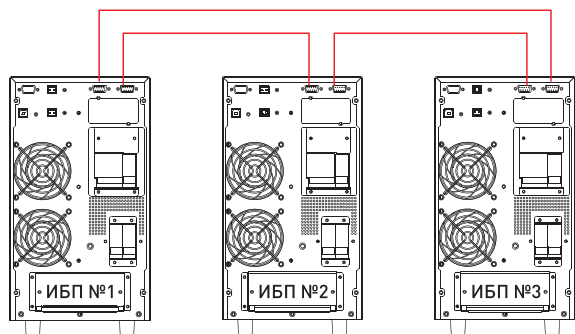
Рисунок 7 – Подключение коммуникационных кабелей 3х ИБП
