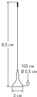
Рис. 1 Антенна WDT 433
