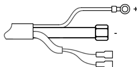
Раздельное подключение
