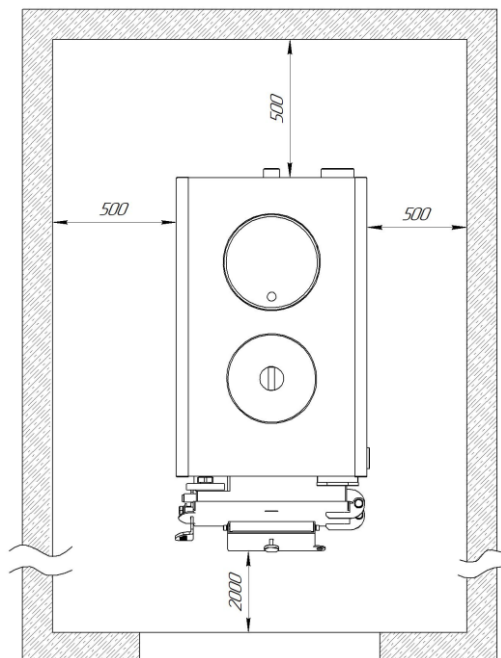
Рисунок 4 – Размещение котла в котельной
