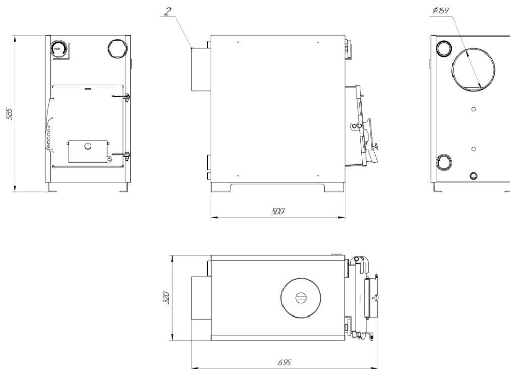
Рисунок 2б – Габаритные размеры и элементы котла «Муравей-10 ГТ» (с горизонтальным дымоходом)
