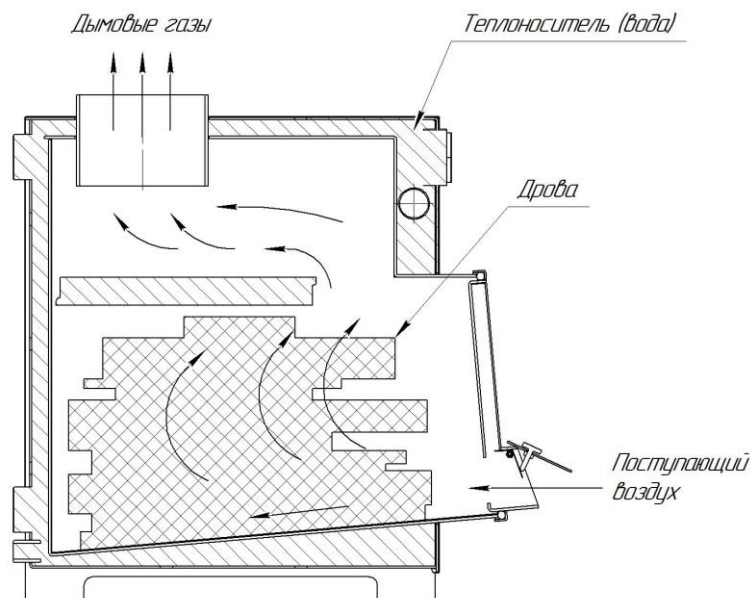
Рисунок 1 - Схема котла «Муравей-10» (с вертикальным дымоходом)
