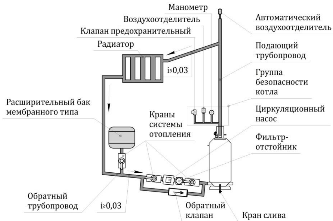
Рисунок 10 – Схема закрытой системы со смешенной циркуляцией
