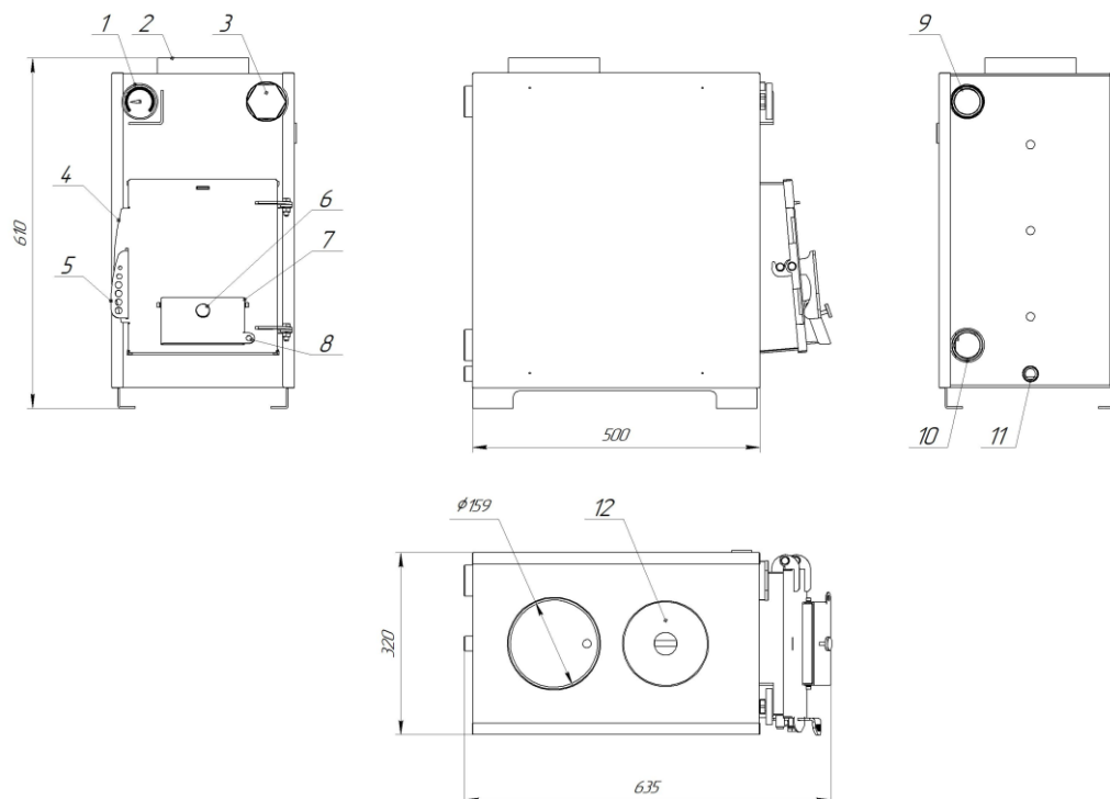
Рисунок 2а – Габаритные размеры и элементы котла «Муравей-10» (с вертикальным дымоходом)
