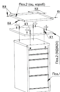
Рис. 4. Крепление Столешницы к Тумбе
