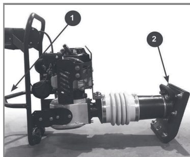
Рис. 20 Транспортирование в горизонтальном положении
