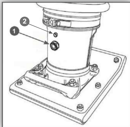
Рис. 6 Проверка уровня масла в рабочем цилиндре
