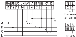
Рисунок 6 – Схема подключения прибора DMC-r
