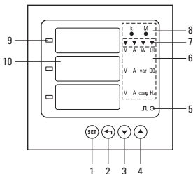
Рисунок 9 – Схема панели управления
