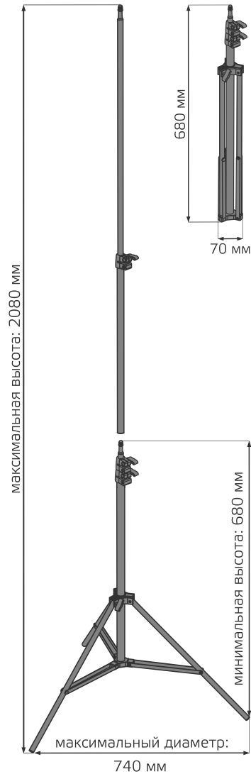
Рис. 1. Возможность регулирования высоты напольной треноги
