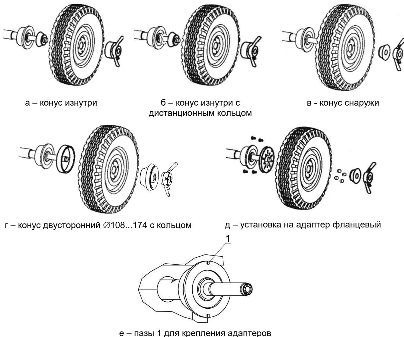
Рисунок 5.3 – Установка колеса
