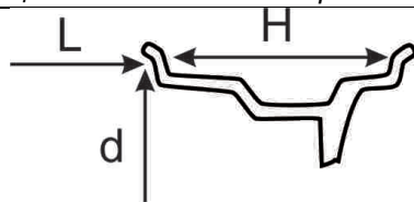
Рисунок 5.4 – Размеры диска
