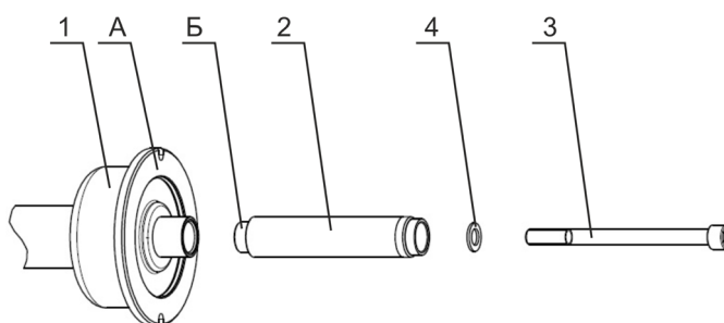
Рисунок 4.2 – Сборка вала
