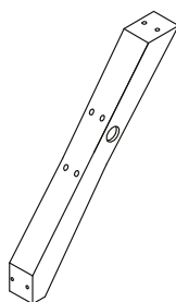
P5 — Левая нога (1 шт).
