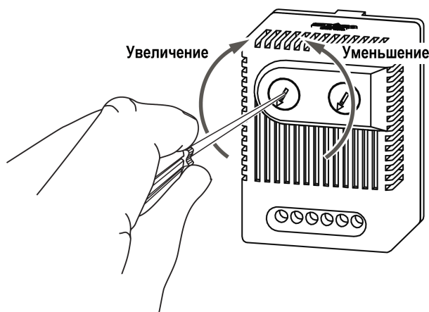
Рисунок 8.1 – Настройка уставки
