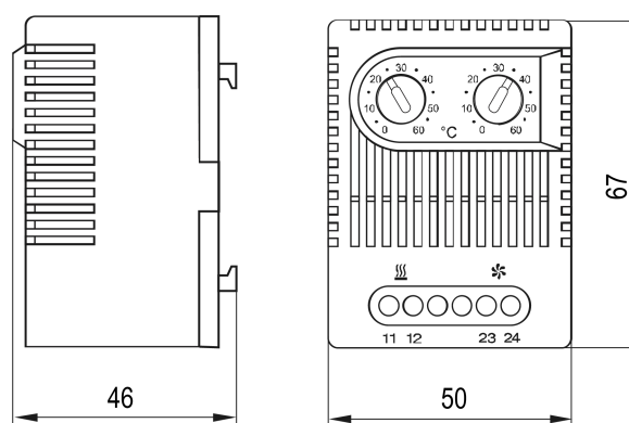
Рисунок 5.3 – Габаритные размеры МТК-СТ2
