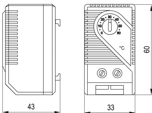
Рисунок 5.2 – Габаритные размеры МТК-СТ0 и МТК-СТ1
