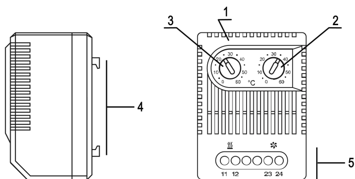
Рисунок 4.2 – Конструкция МТК-СТ2
