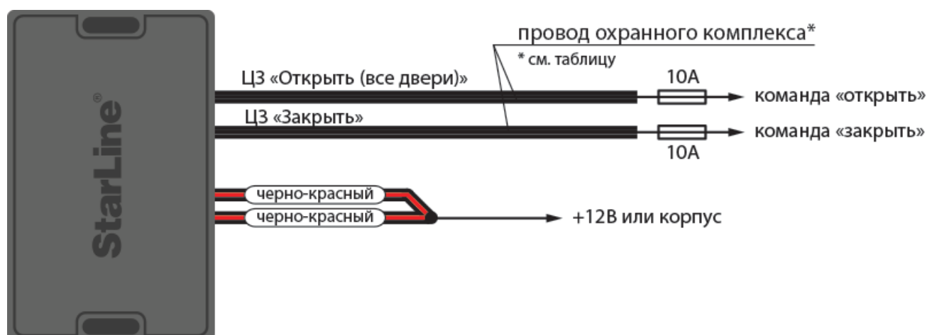
Схема аналогового подключения центрального замка с положительным или отрицательным силовым управлением для охранных комплексов StarLine A96/A66, B96/B66, D96/D66, AS96 (v2)
