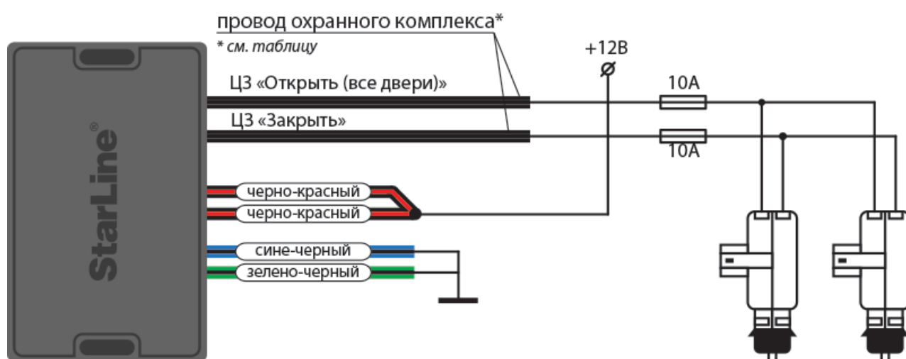
Схема аналогового подключения центрального замка к двухпроводным приводам для охранных комплексов StarLine A96/A66, B96/B66, D96/D66, AS96 (v2)
