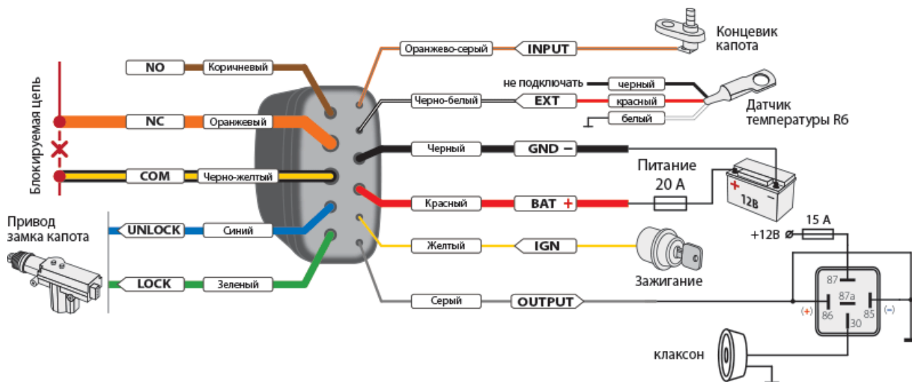
Рис. 3. Схема подключения сирены, управляемой подкапотным блоком StarLine R6
