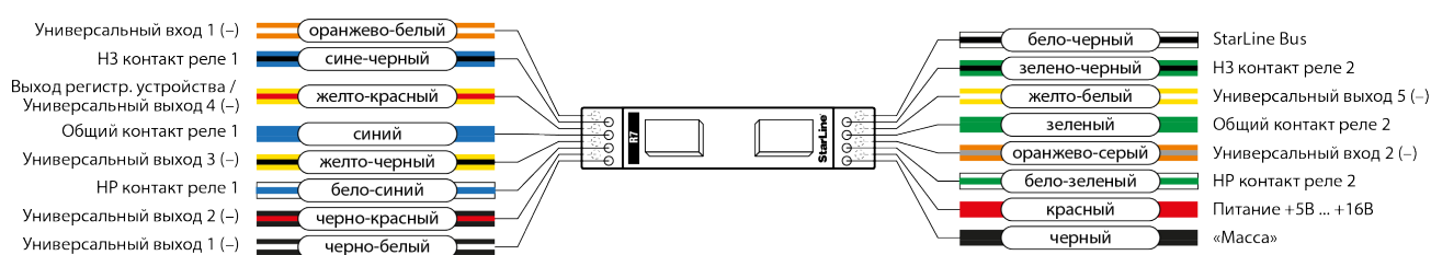
Рис. 6. Схема подключения кодового многоканального микрореле StarLine R7
