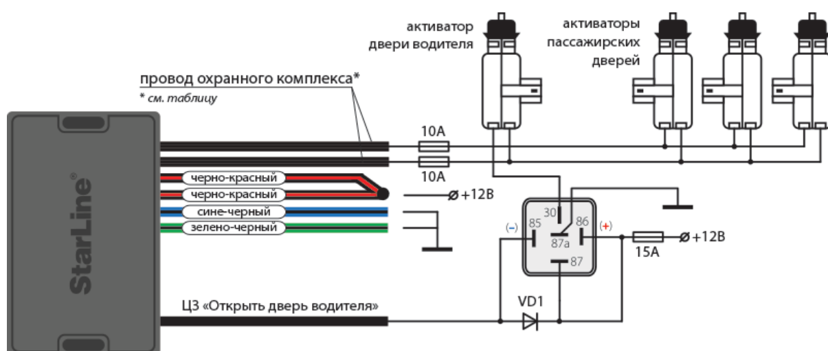
Рис. 4. Схема подключения к двухпроводным приводам системы запирания для последовательного отпираания замков дверей
