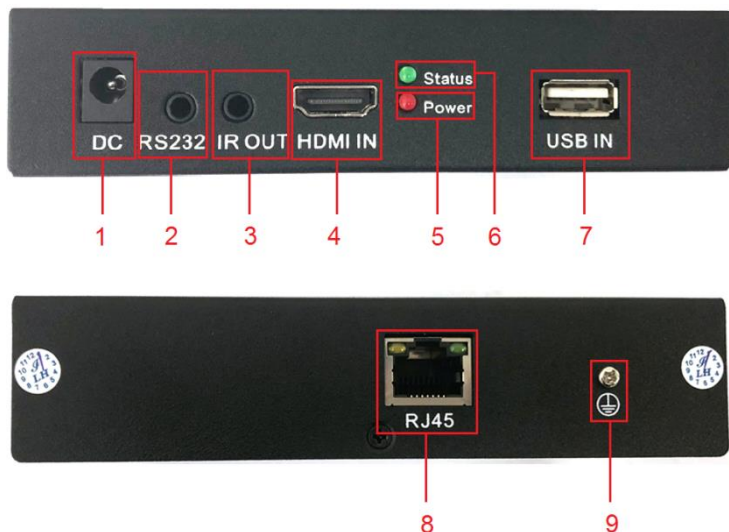
Рис. 2 Передатчик TLN-HiKM/1(ver.2), разъемы и индикаторы передней и задней панели
