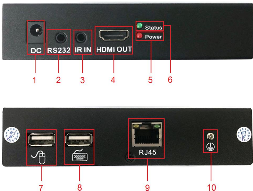
Рис. 3 Приемник RLN-HiKM/1(ver.2), разъемы и индикаторы передней и задней панели
