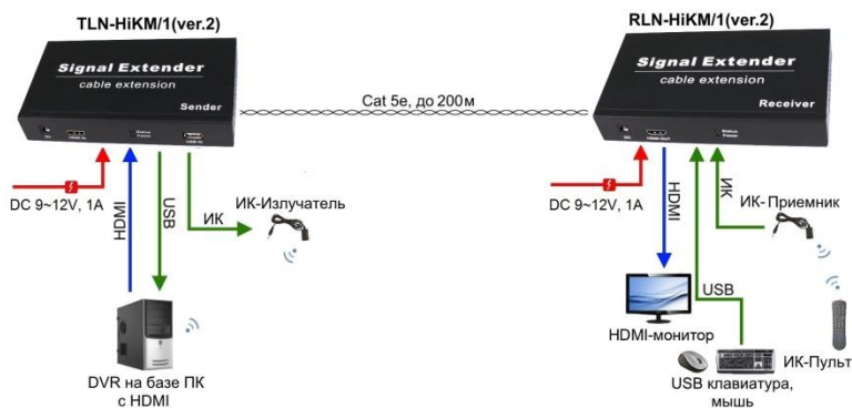
Рис.5 Схема подключения комплекта TLN-HiKM/1+RLN-HiKM/1(ver.2) в режиме «точка – точка».
