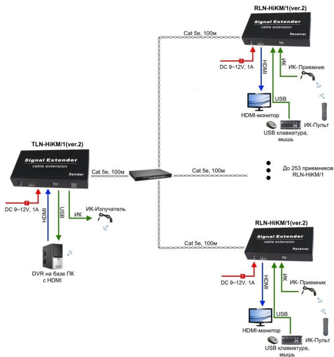
Рис.4 Схема подключения комплекта TLN-HiKM/1+RLN-HiKM/1(ver.2) в режиме «точка – многоточка».
