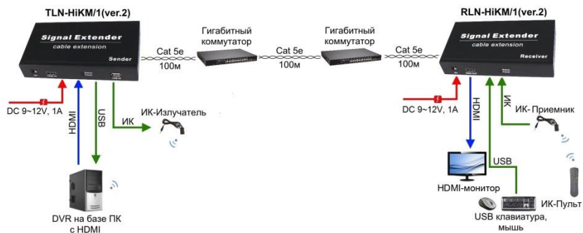
Рис.6 Схема подключения комплекта TLN-HiKM/1+RLN-HiKM/1(ver.2) в режиме «точка – точка» через коммутатор без ограничения по количеству.
