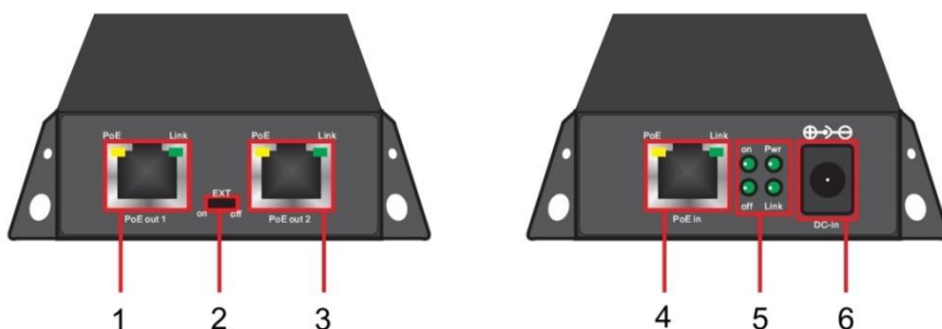
Рис. 3 Панели подключения коммутатора/удлинителя SW-8030/D
