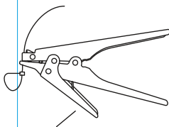
Рисунок 4 – Обрезка кабельного хомута нажимной рукояткой
