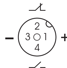
Цоколевка соединителя (вид со стороны монтажа)
