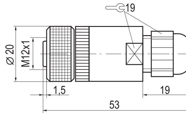
Габаритный чертеж
