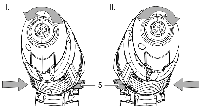
I. Вкручивание винтов II. Выкручивание винтов
