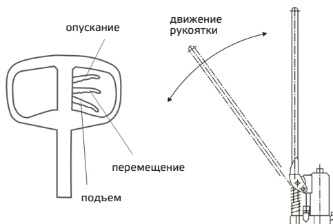
Рисунок 6. Рабочие режимы рычага управления
