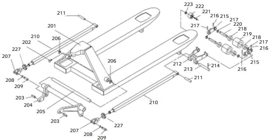
Рисунок 3. Состав корпуса гидравлической тележки PROLIFT PRO/RT
