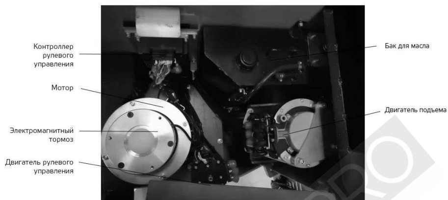
Рисунок 5. Расположение основных деталей
