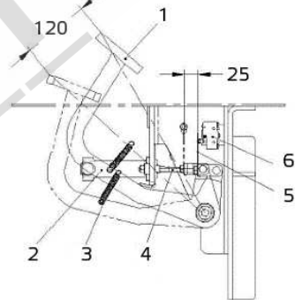
Рисунок 17. Строение педали тормоза
