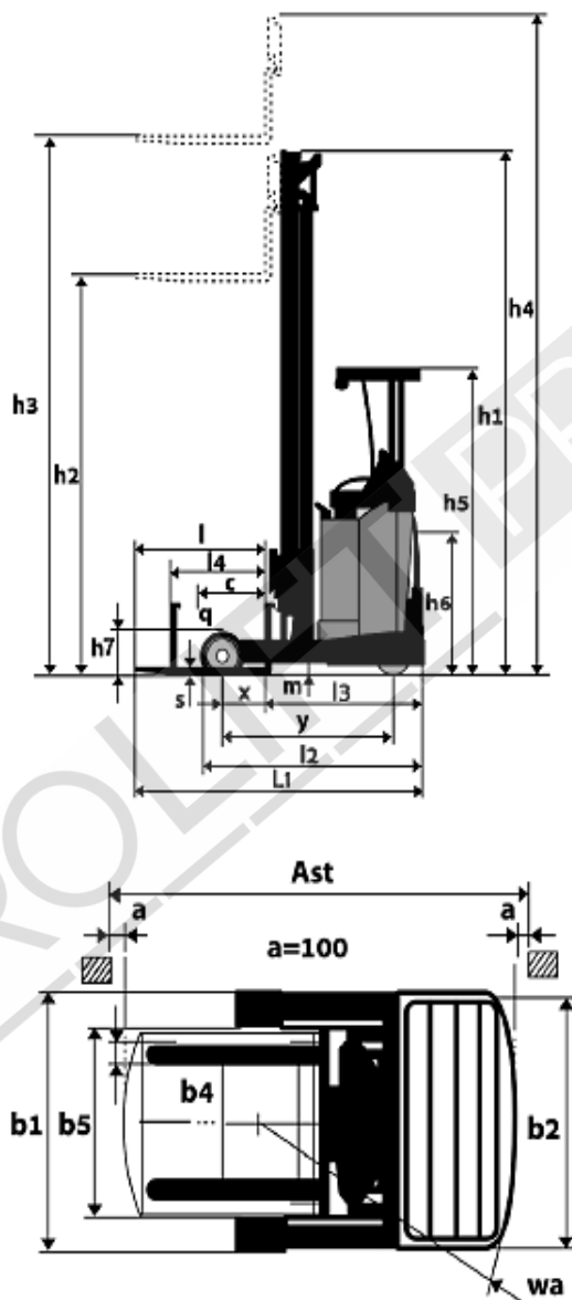
Рисунок 1. Технические характеристики ричтрака
