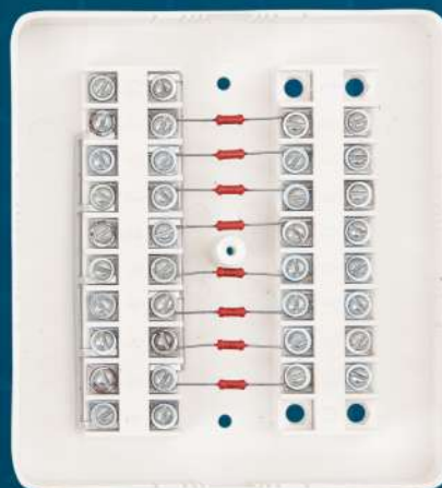
КРА-4 (75 Ом)
