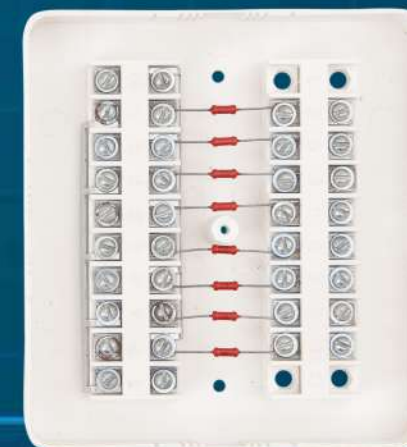
КРА-4 (300 Ом)
