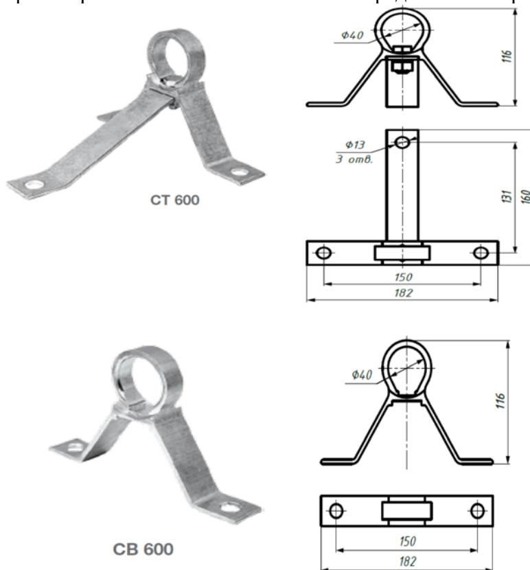
Рис. 1. Внешний вид анкерных кронштейнов СТ 600 и СВ 600.
