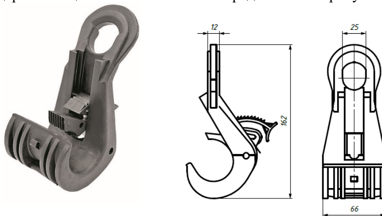
Рис. 1. Внешний вид поддерживающего зажима PS 16/120.
