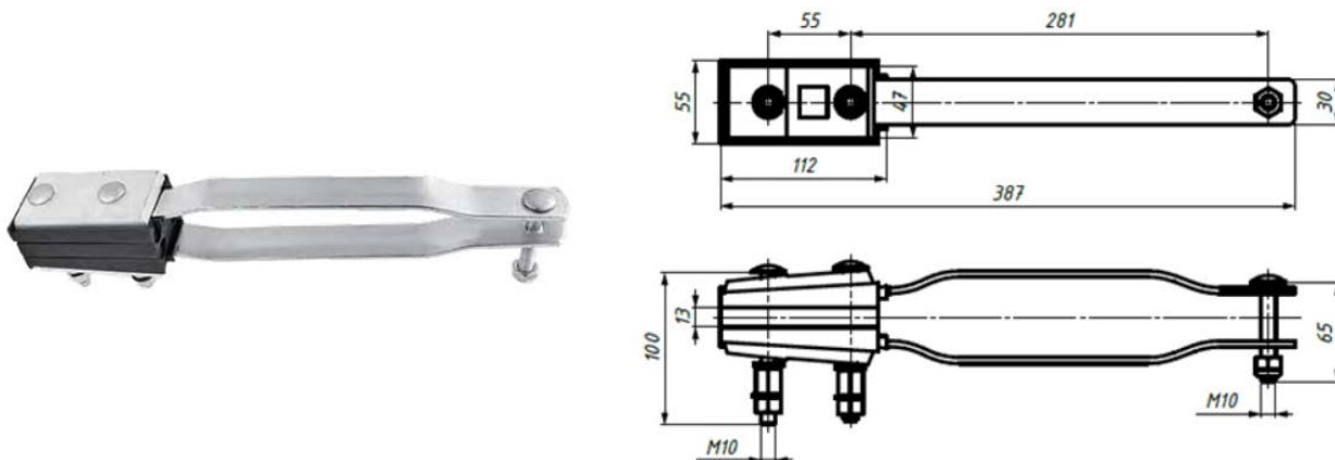
Рис. 1. Внешний вид анкерного зажима RPA 450/120.S.
