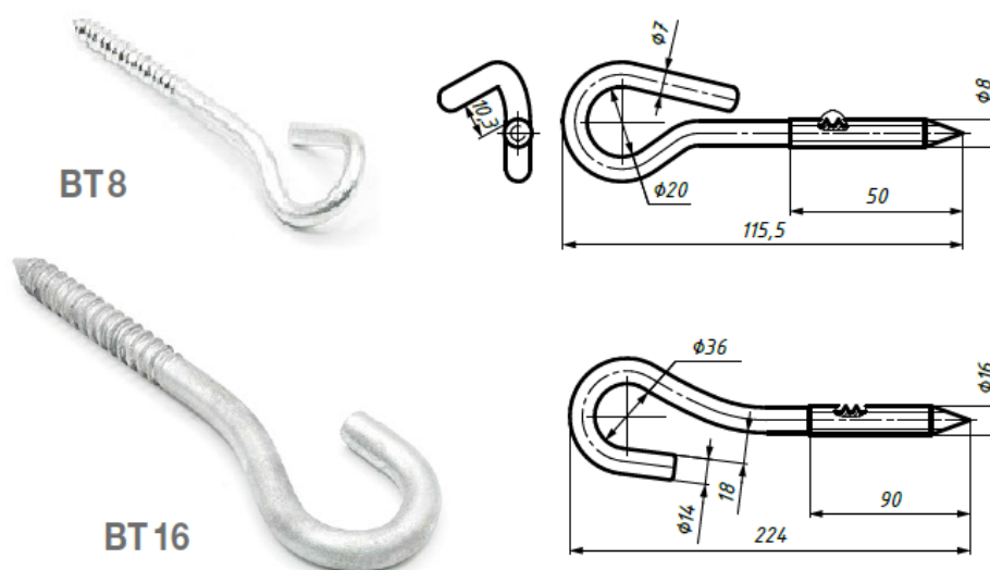
Рис. 1. Внешний вид крюков-шурупов ВТ 8 и ВТ 16.
